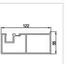
Weight: 2.734kg/m Thickness: mm 型号：GM-013 名称：榫卯副梁 重量：2.734kg/m 壁厚：mm
