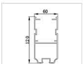
Weight: 2.186kg/m Thickness: 1.8mm 型号：GM-002 名称：120主梁 重量：2.186kg/m 壁厚：1.8mm
