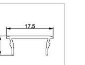
型号：GM-168-232 名称：120阳光房压型 重量：0.073kg/m 壁厚：1.0mm
