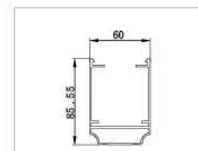
Weight: 1.526kg/m Thickness: 1.6mm 型号：GM-004 名称：85副梁 重量：1.526kg/m 壁厚：1.6mm
