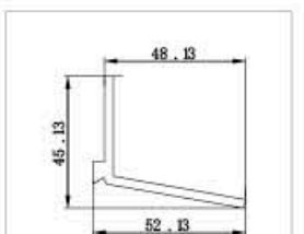
型号：GM-007 名称： 重量：0.743kg/m 壁厚：3.0mm
