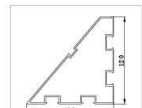
型号：GM-006 名称：120三角梁 重量：2.48kg/m 壁厚：1.8mm
