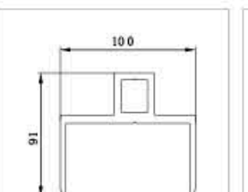
型号：HQ-2841 名称： 重量：4.001kg/m 壁厚：4.0mm
