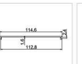
型号：GM-009 名称：120立柱盖 重量：0.518kg/m 壁厚：mm
