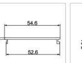
型号：GM-168-267A 名称：靠墙梁盖 重量：0.168kg/m 壁厚：1.0mm
