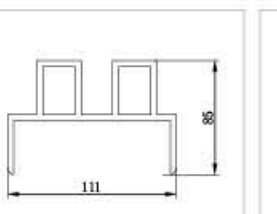
型号：GM-906 名称： 重量：4.525kg/m 壁厚：mm
