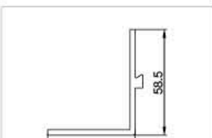
型号：GM-014 名称： 重量：0.918kg/m 壁厚：3.0mm
