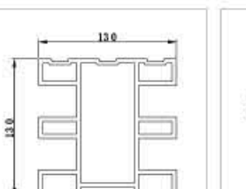
型号：GM-905 名称： 重量：9.72kg/m 壁厚：mm
