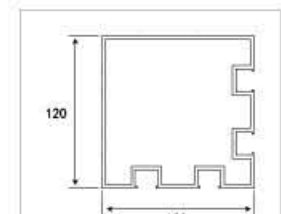
型号：GM-168-264 名称：120立柱 重量：4.58kg/m 壁厚：3.0mm
