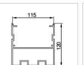
Weight: 4.486kg/m Thickness: 2.85mm 型号：GM-010A-3.0 名称： 重量：4.486kg/m 壁厚：2.85mm
