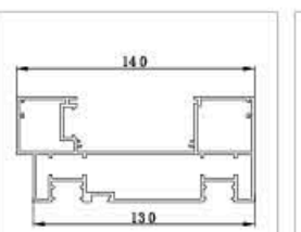
型号：GM-001 名称：灯带外框 重量：3.13kg/m 壁厚：1.8mm
