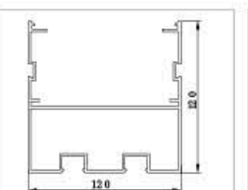
Weight: 3.016kg/m Thickness: 1.8mm 型号：GM-010 名称：120立柱 重量：3.016kg/m 壁厚：1.8mm
