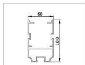
Weight: 1.99kg/m Thickness: 1.8mm 型号：GM-003 名称：100副梁 重量：1.99kg/m 壁厚：1.8mm
